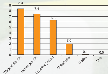
Durchschnittlicher Energieverbrauch pro 100 km (in l Benzin gerechnet)
